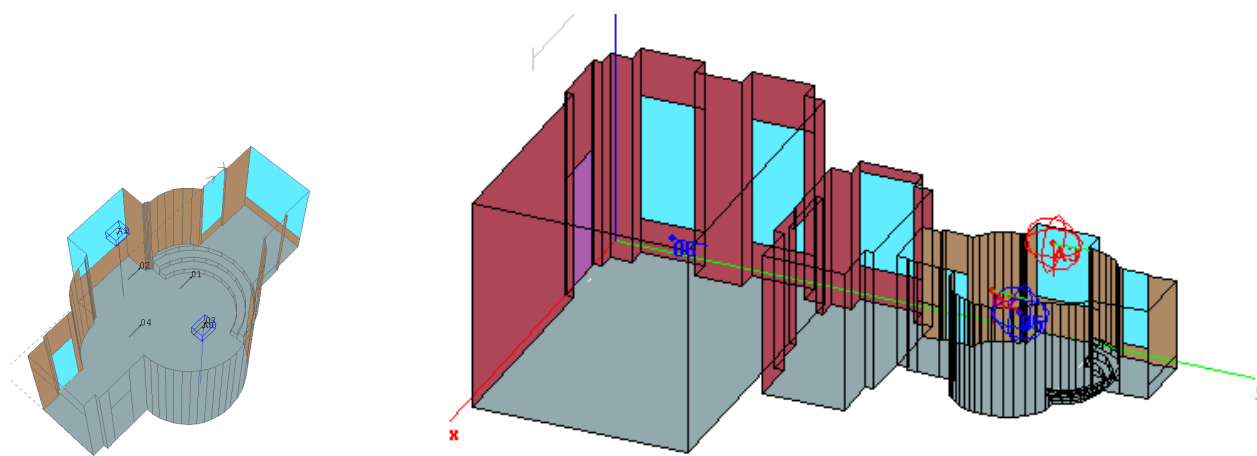
Simulation CATT Acoustique Salle des Pas Perdus
